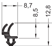
Уплотнение коробки EPDM
