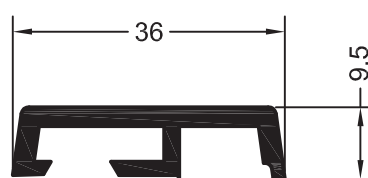
Наличник для окна со штульпом
