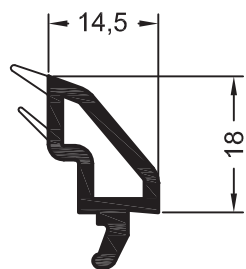
Штапик Softline 14,5 561145 @ 144 597145 @ 72
