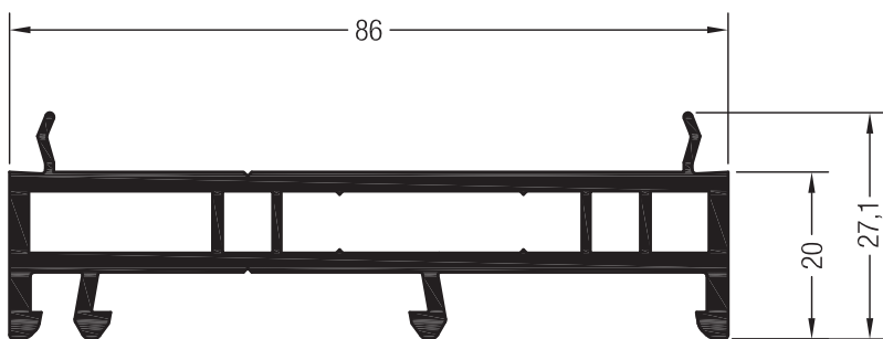
Профиль доборный 20/86
