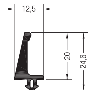
Уплотнение центральное PREN
