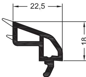
Штапик Softline 22,5 550120 @ 144 599120 @ 72
