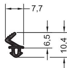
Уплотнение притвора Z PREN
