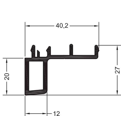
Профиль подставочный 38
