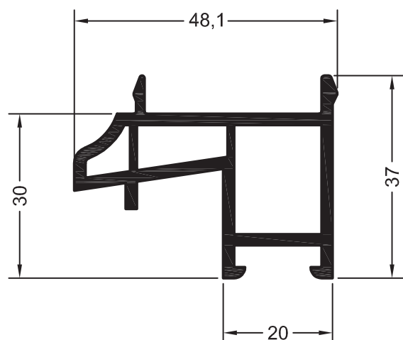
Профиль подставочный 42
