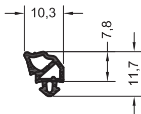
Уплотнение универсальное PREN
