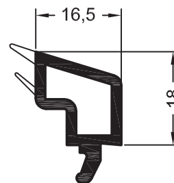
Штапик 16,5
