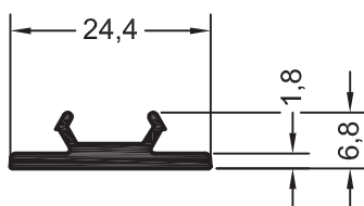
Заглушка фурнитурного паза 24
