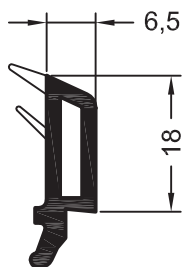
Штапик 6,5
