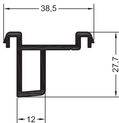
Профиль подставочный ремонтный
