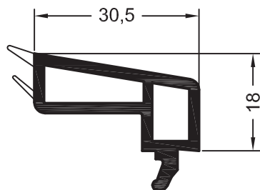
Штапик 30,5
