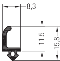
Уплотнение для штульпа GENEEO
