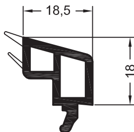
Штапик 18,5
