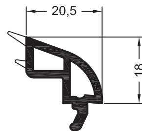
Штапик закругленный 20,5
