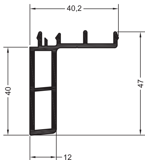
Профиль подставочный 40
