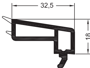
Штапик 32,5
