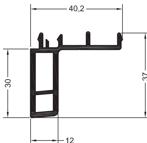
Профиль подставочный 39
