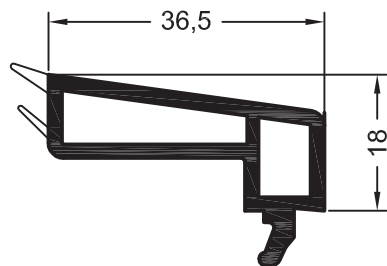
Штапик 36,5
