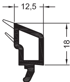
Штапик 12,5
