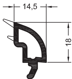
Штапик закругленный 14,5
