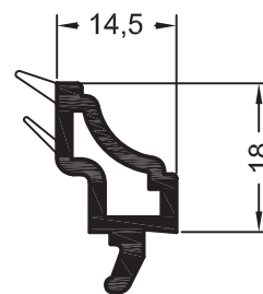
Штапик фигурный 14,5 561850 @ 144
