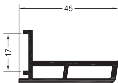
Нащельник 45
