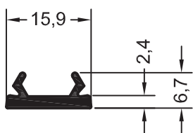
Заглушка фурнитурного паза 16
