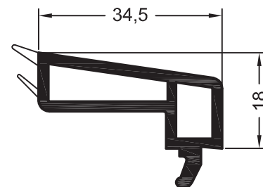
Штапик 34,5
