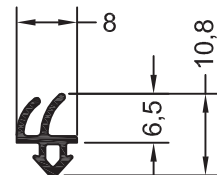
Уплотнение притвора EPDM
