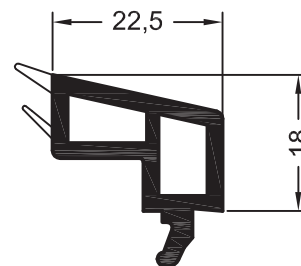
Штапик 22,5
