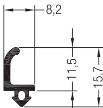
Уплотнение для штульпа ED86
