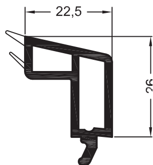
Штапик 22,5 для глухого остекления
