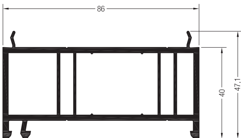
Профиль доборный 40/86
