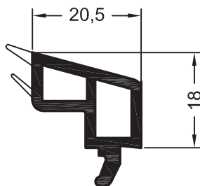
Штапик 20,5
