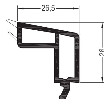
Штапик 26,5 для глухого остекления
