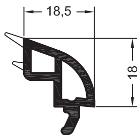
Штапик закругленный 18,5
