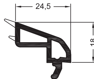
Штапик Softline 24,5 541043 144
