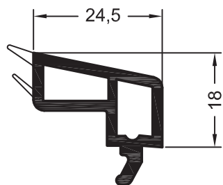
Штапик 24,5
