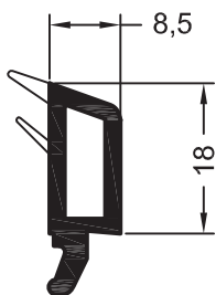
Штапик 8,5
