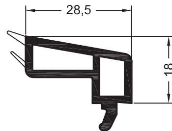
Штапик 28,5
