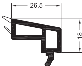
Штапик 26,5
