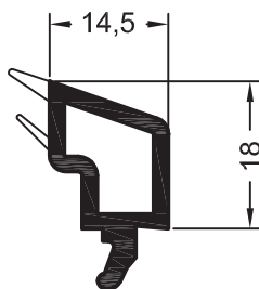
Штапик 14,5
