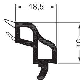
Штапик декоративный 18,5 543211 @ 573211 @ 36
