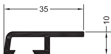
Наличник 35
