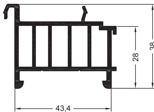
Профиль подставочный 30/43
