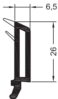
Штапик 6,5 для глухого остекления
