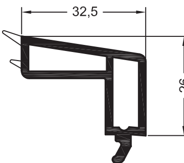
Штапик 32,5 для глухого остекления
