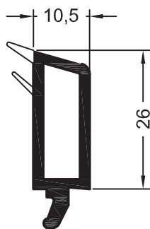
Штапик 10,5 для глухого остекления
