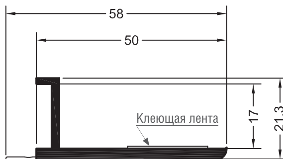
Нащельник 50
