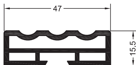
Профиль декоративный 1
