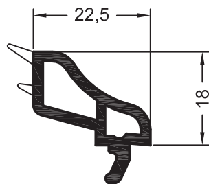
Штапик декоративный 22,5 561073 144 597073 @ 72
