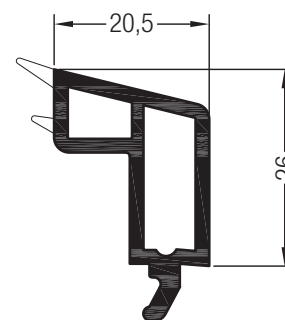
Штапик 20,5 для глухого остекления
