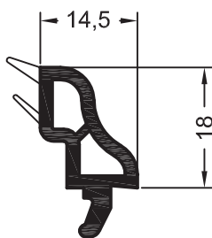
Штапик декоративный 14,5 561620 @ 144 596930 @ 72
