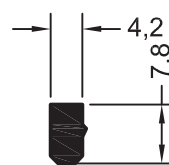
Профиль-заглушка паза штапика
