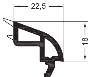
Штапик закругленный 22,5
