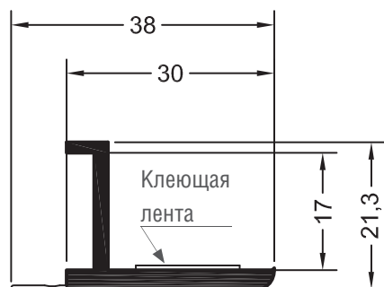
Нащельник 30
