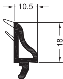
Штапик декоративный 10,5 561720 @ 144 597070 @ 72
