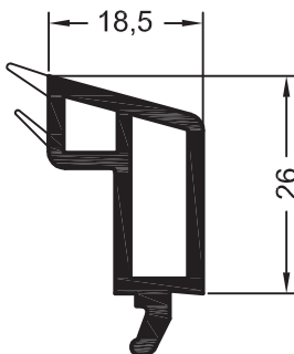
Штапик 18,5 для глухого остекления
