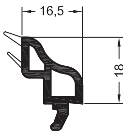
Штапик декоративный 16,5 543371 @ 573371 @ 144
